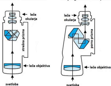
Slika 1: Struktura daljnogleda s Porro in strešno prizmo
